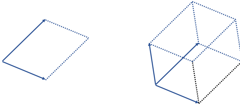
图 7.5: DPP 几何结构示意图。
